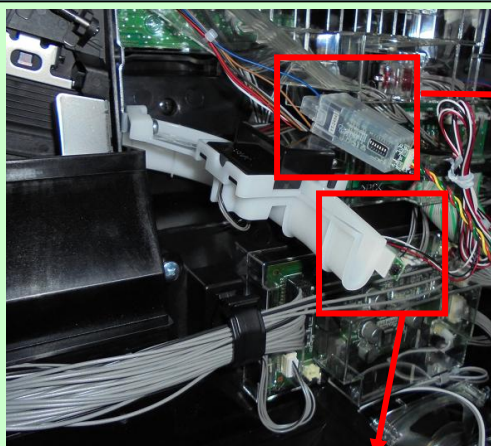
反射センサー取付例
