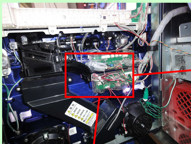
電流センサー取付例
