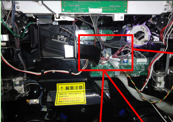
反射センサー取付例
