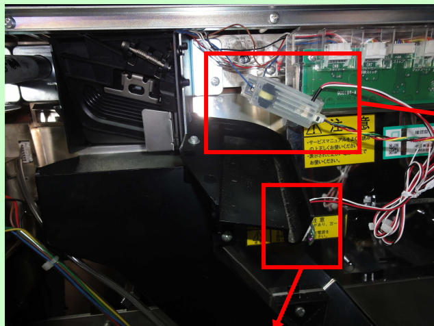
反射センサー取付例
