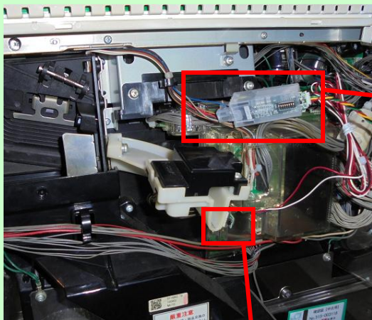
反射センサー取付例
